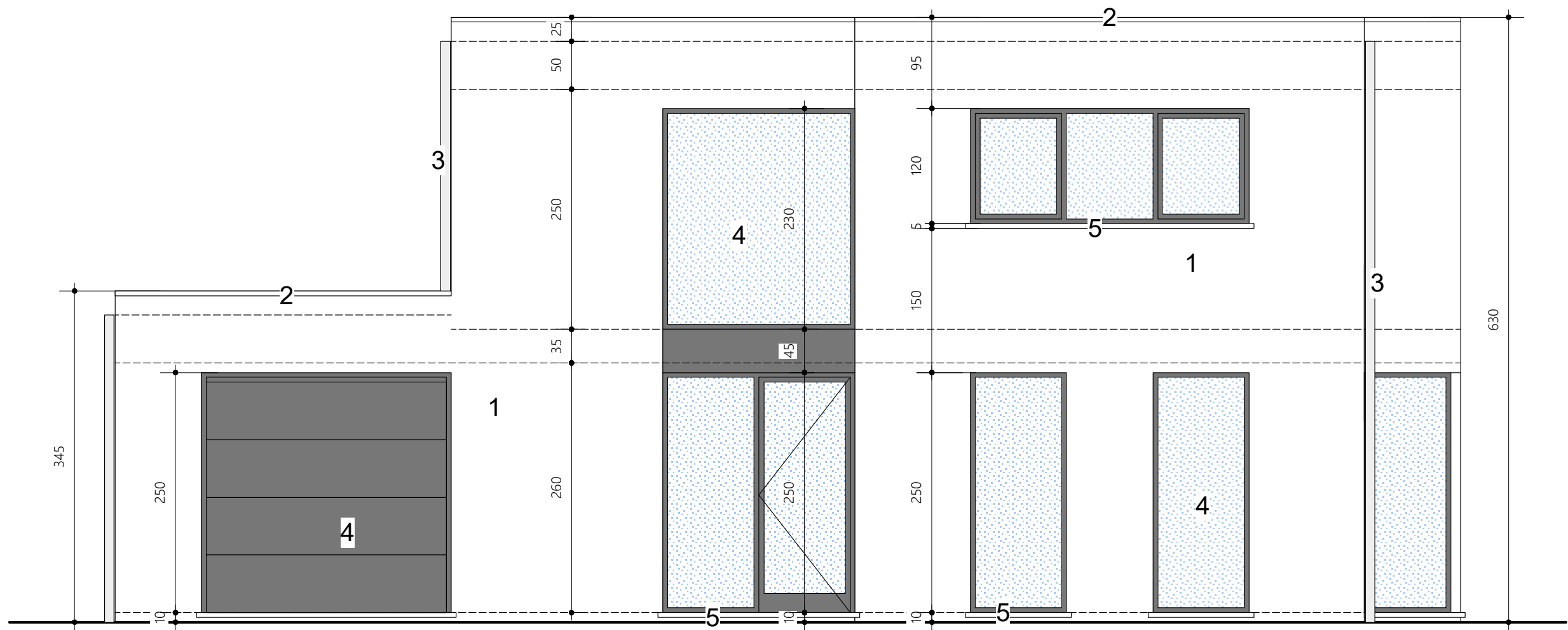
vooraanzicht 1/50
