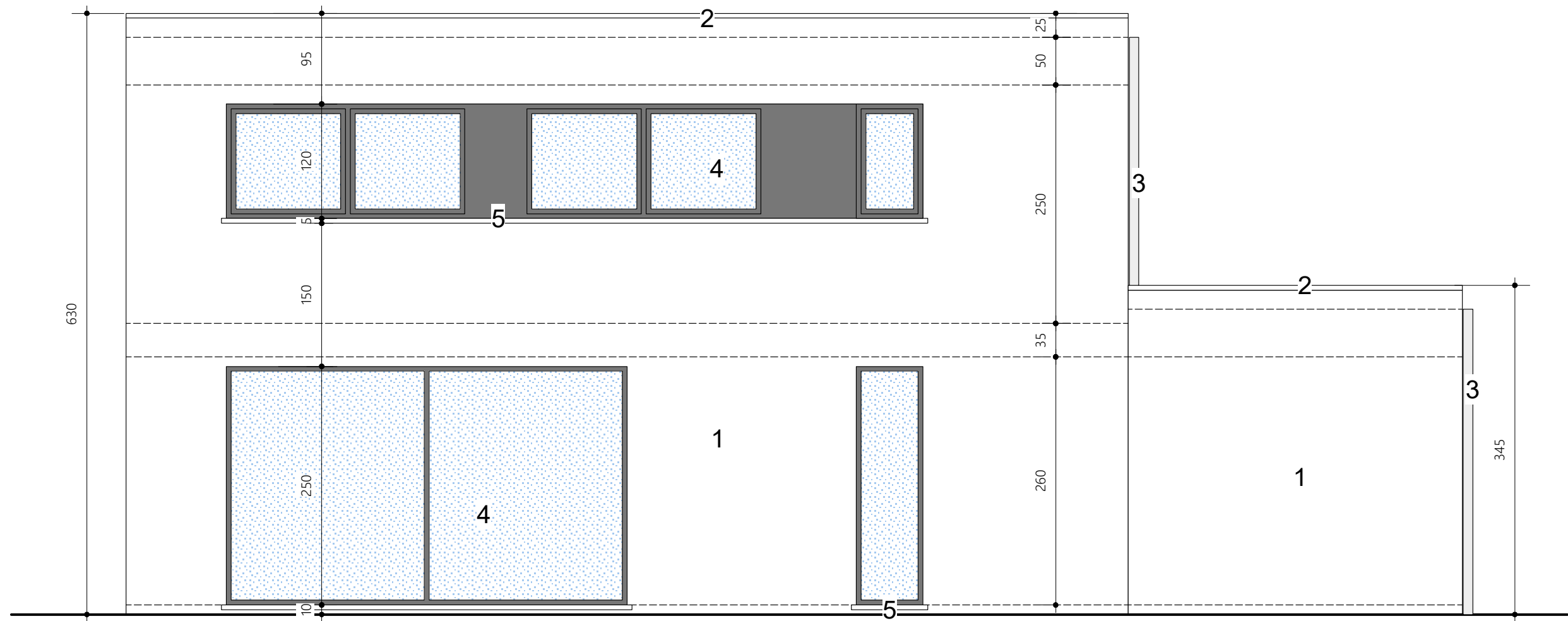
achteraanzicht 1/50
