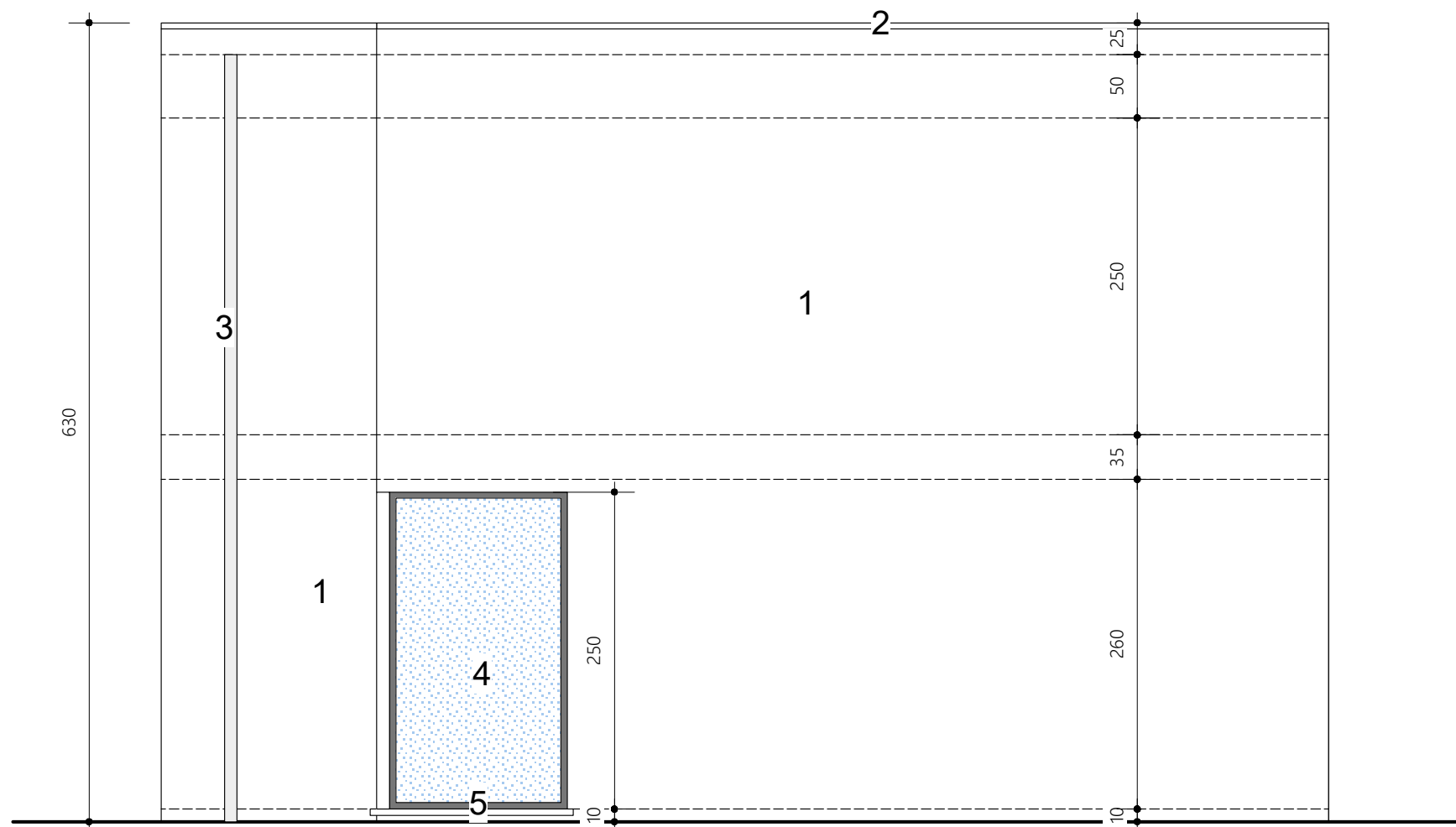
rechteraanzicht 1/50
